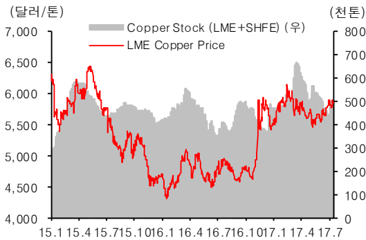
도표 5 전기동 가격 및 재고 추이
