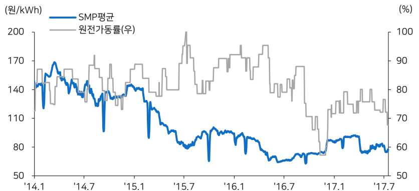
[Key Chart] 원전가동률 대비 SMP 주간평균 추이
