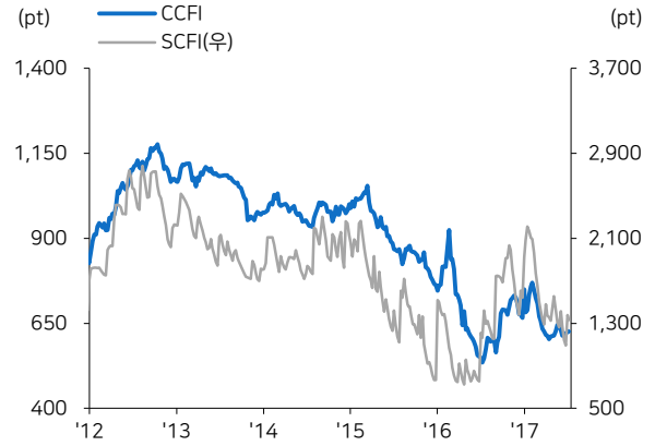
그림20 미주노선(W/C) CCFI, SCFI
