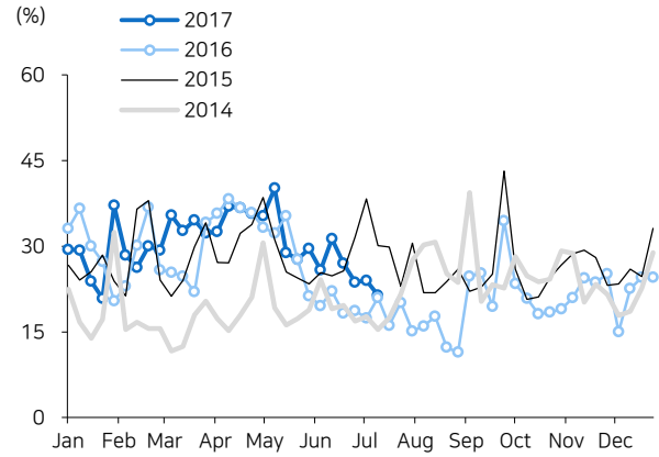
그림2 주간 평균 전력공급 예비율
